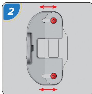
Réglage horizontal de la gâche
