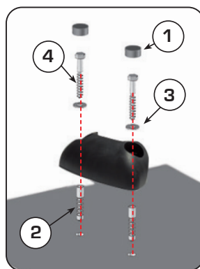
Fixation du sabot
