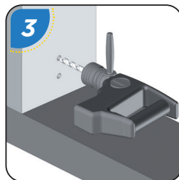
Perçages \varnothing 14
